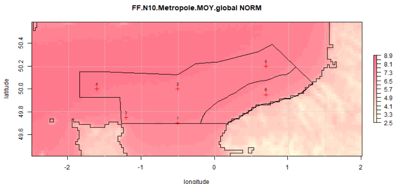
Illustration 2: Vent moyen à 10 m d'altitude (m/s) sur la macrozone Normandie
