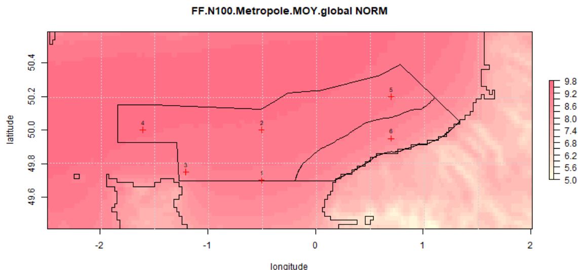
Illustration 1: Vent moyen à 100 m d'altitude (m/s) sur la macrozone Normandie
